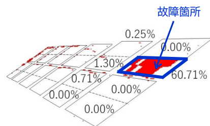
図7 温度上昇の二値化画像
