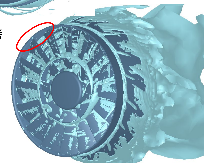
図3 羽根車まわりの流れ場予測結果
