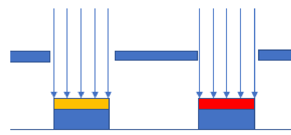
イオン注入
