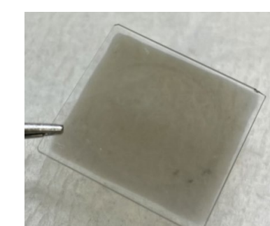
MoS 2 薄膜
